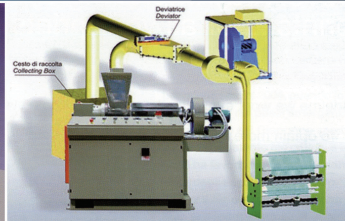
estrusore per recupero rifili da linee blow film
