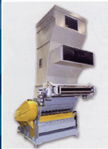
mulino per film-linee: cast e blow film con tramo recupero bobine
