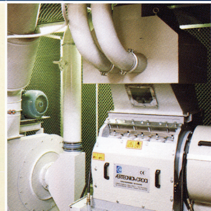
gruppo macinazione rifili
